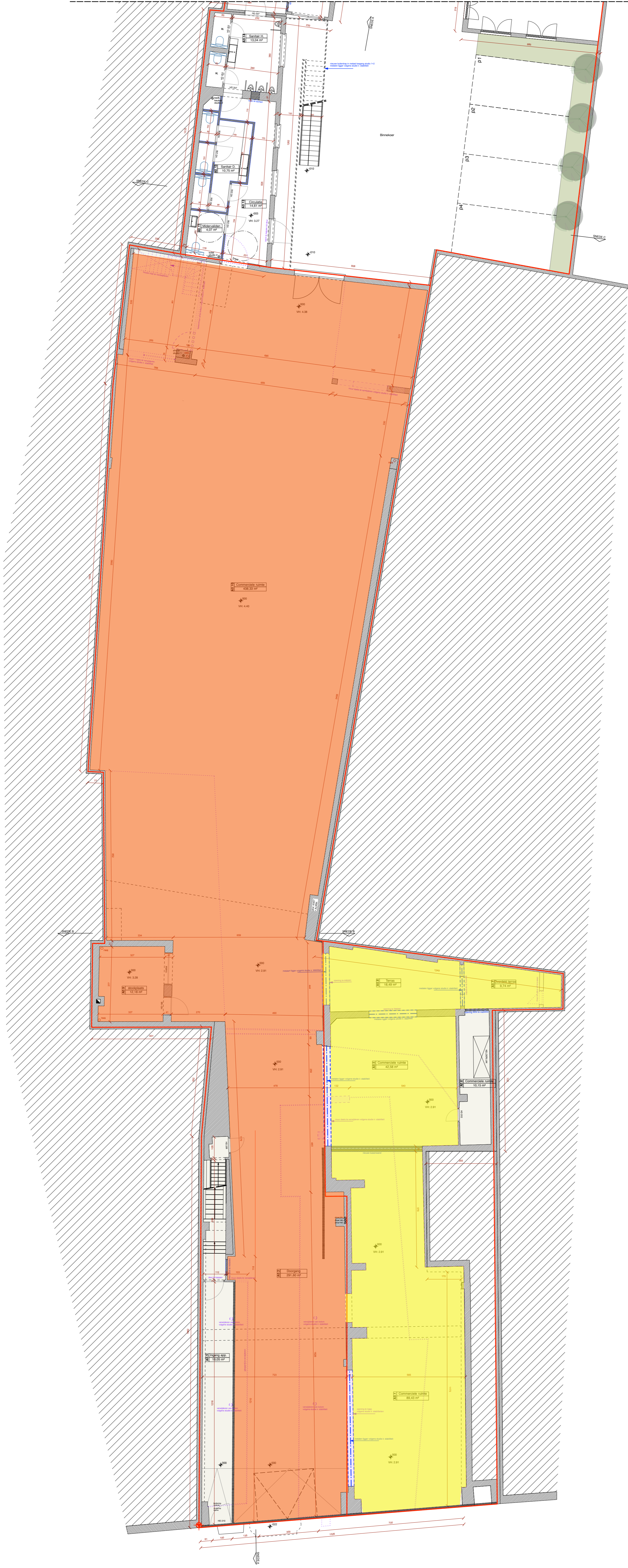
gelijkvloerse verdieping - schaal 1:100 nieuwe toestand
